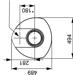
Dopływ powietrza z zewnątrz – podłączenie przez otwór w podłodze, Ø 100mm
