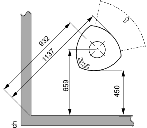
Minimalne odległości od ścian z materiałów palnych
